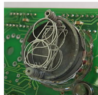
Внутреннее устройство газоразрядного индикатора
