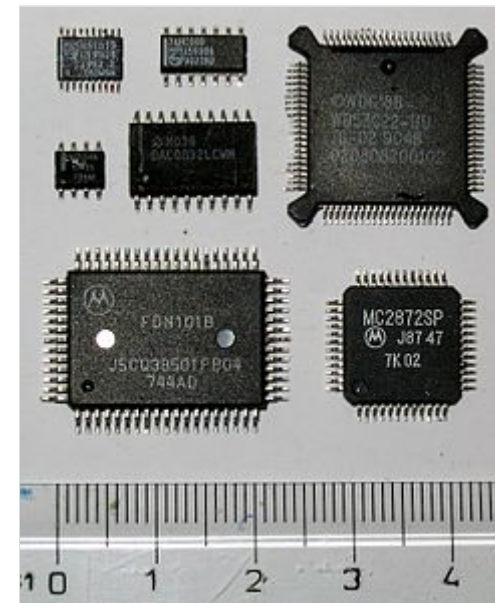
Корпуса интегральных микросхем, предназначенные для поверхностного монтажа
