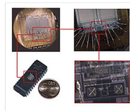
Увеличенное изображение кристалла EPROM 27C512
